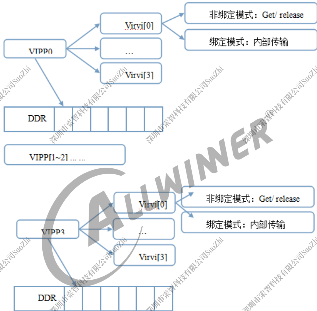
图 3-1: VIPP 非绑定情况
