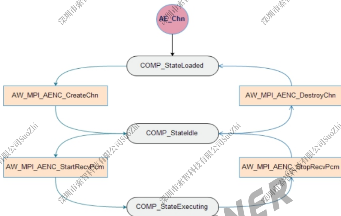
图 9-5: AEnc 通道状态图
