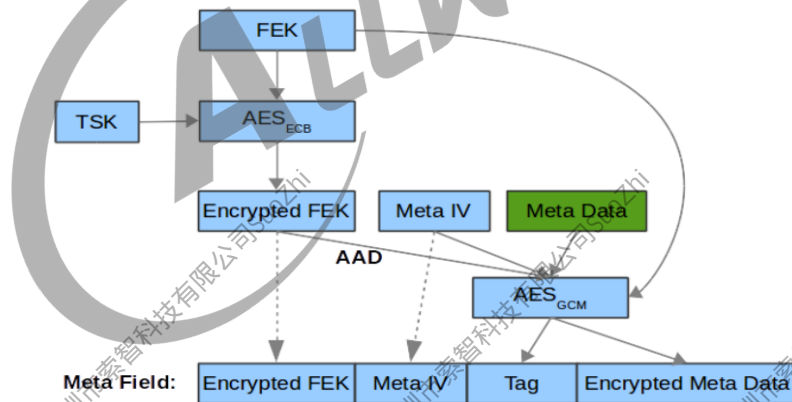
图 6-6: Meta Data 加密流程
