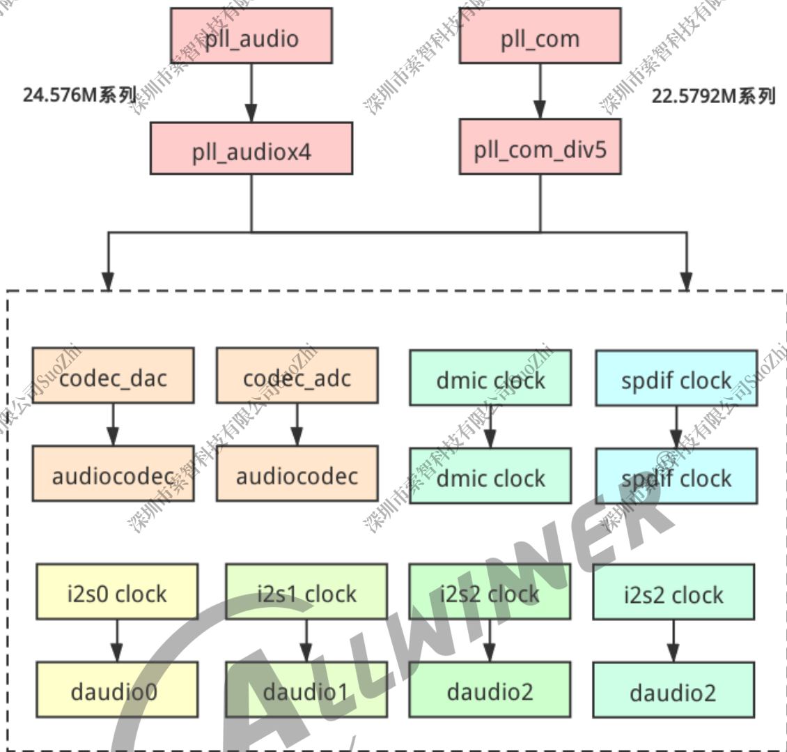
图 2-45: R818 时钟源
