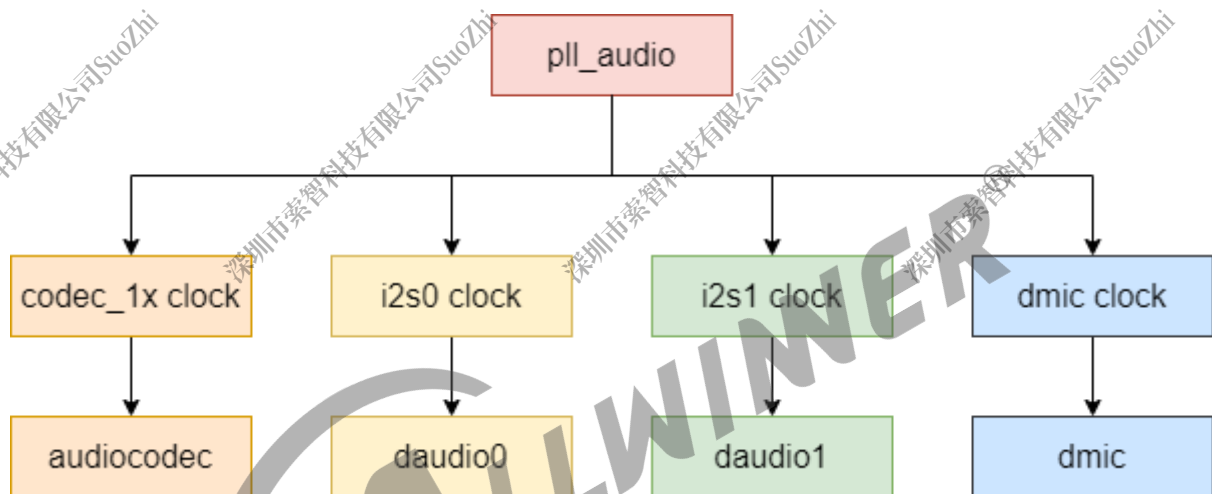
图 2-48: V853 时钟源
