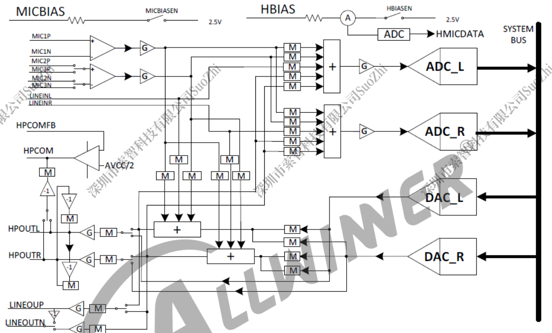
图 2-24: R332 音频通路
