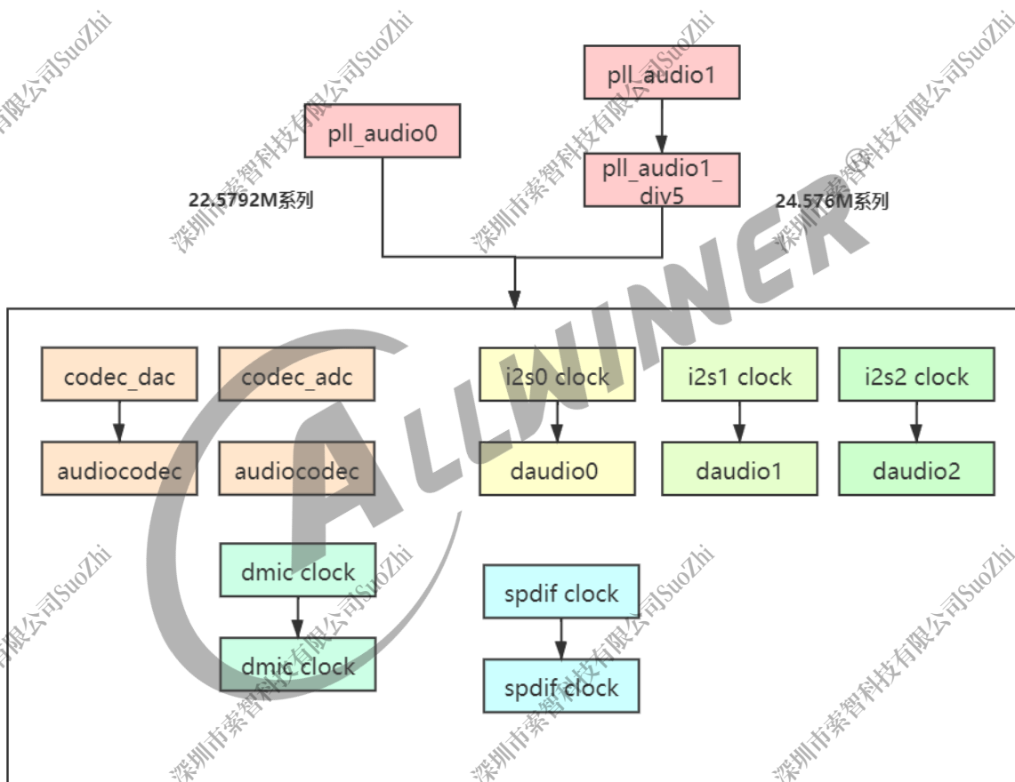
图 2-47: R528 时钟源
