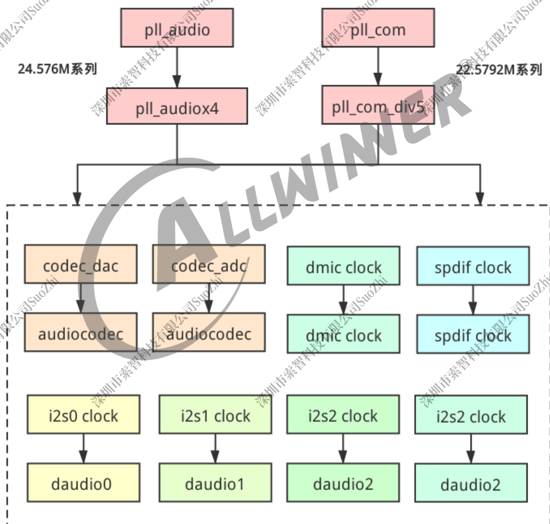
图 2-43: MR813 时钟源
