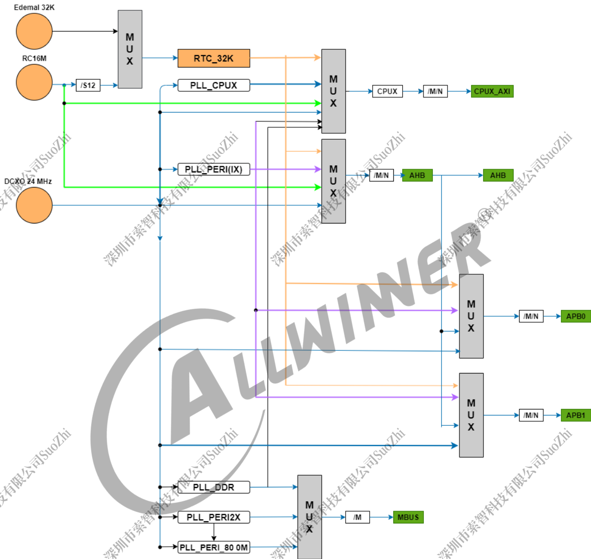
图 1-6: V85x-clk-tree
