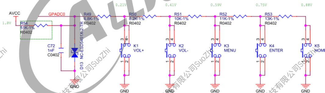
图 2-1: GPADC0
